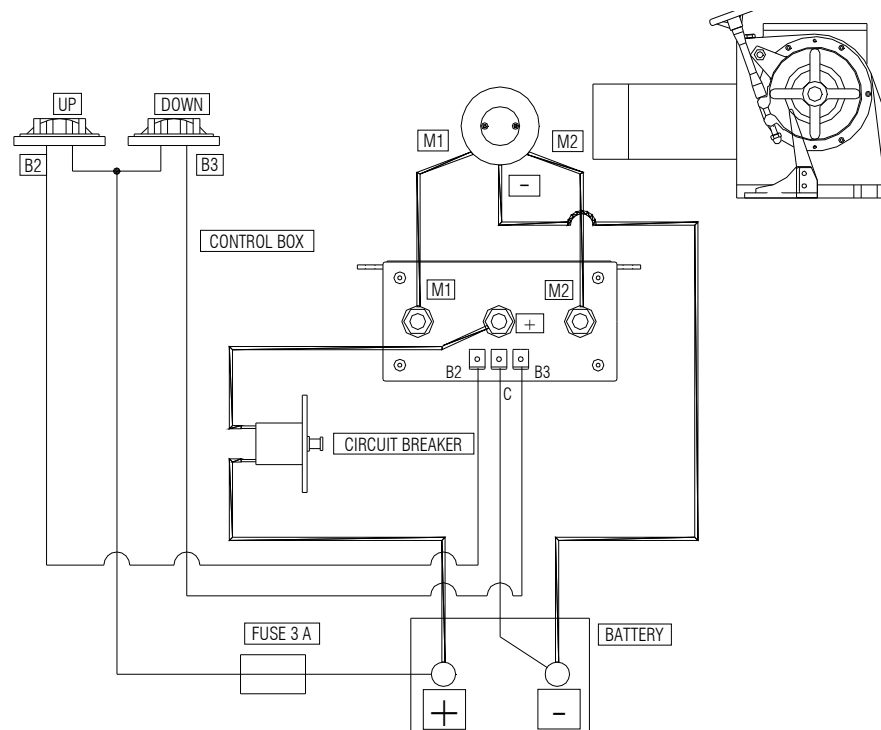
3 terminals motor :
