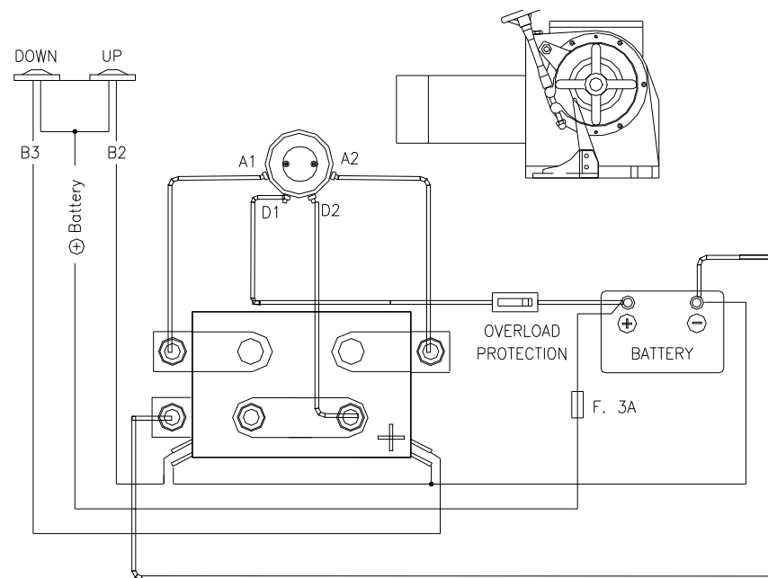
4 terminals motor :
