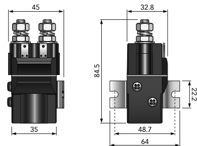
Dimensioni (mm) Dimensions - Dimensions - Abmessungen - Dimensiones
