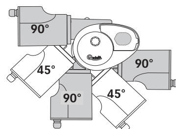
Motoriduttore 1500W
