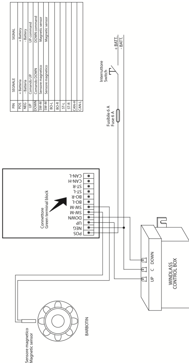
SCHEMA ELETTRICO / ELECTRICAL DRAWING Sensore magnetico reed (2 fili) / Reed magnetic sensor (2 wires)
