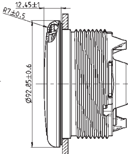
Round bezel
