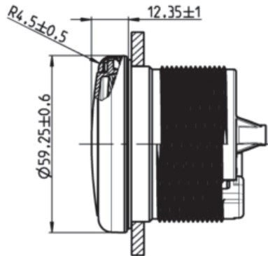
Round bezel
