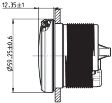
Flat bezel
