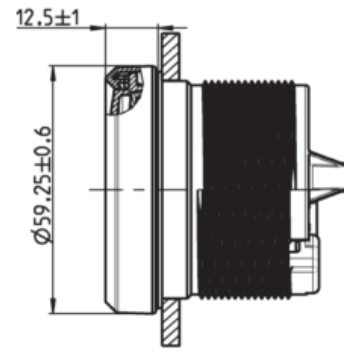
Triangle bezel
